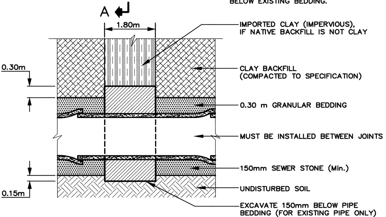
VIEW A-A
