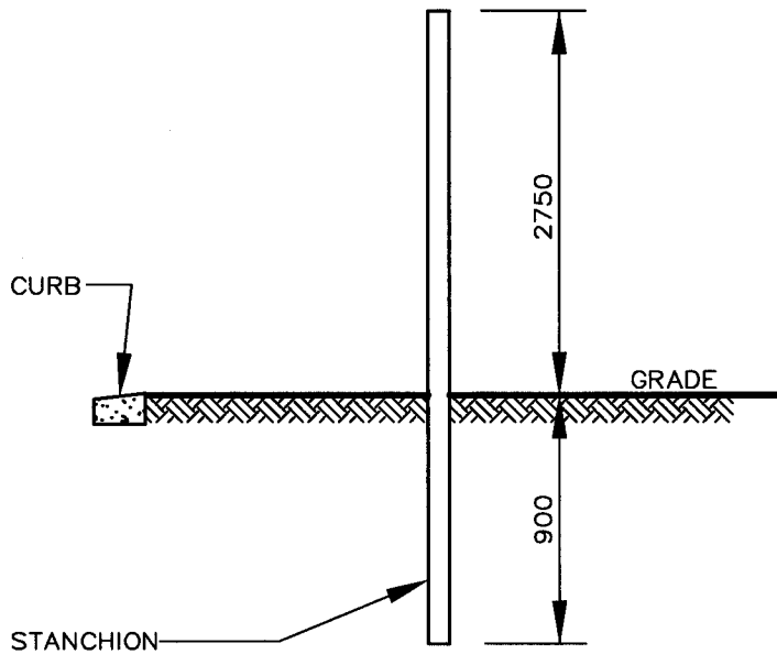
FIG. 1 - BOULEVARD AREAS N.T.S.
