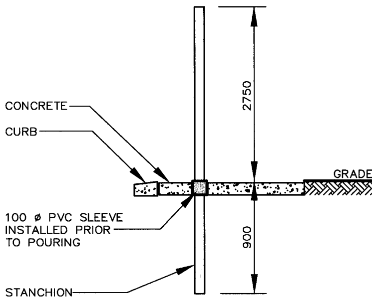
FIG. 2 - CONCRETE AREAS N.T.S.
