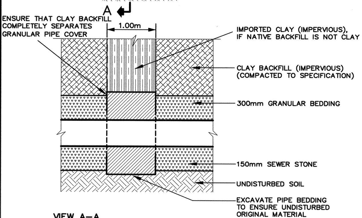
VIEW A-A
